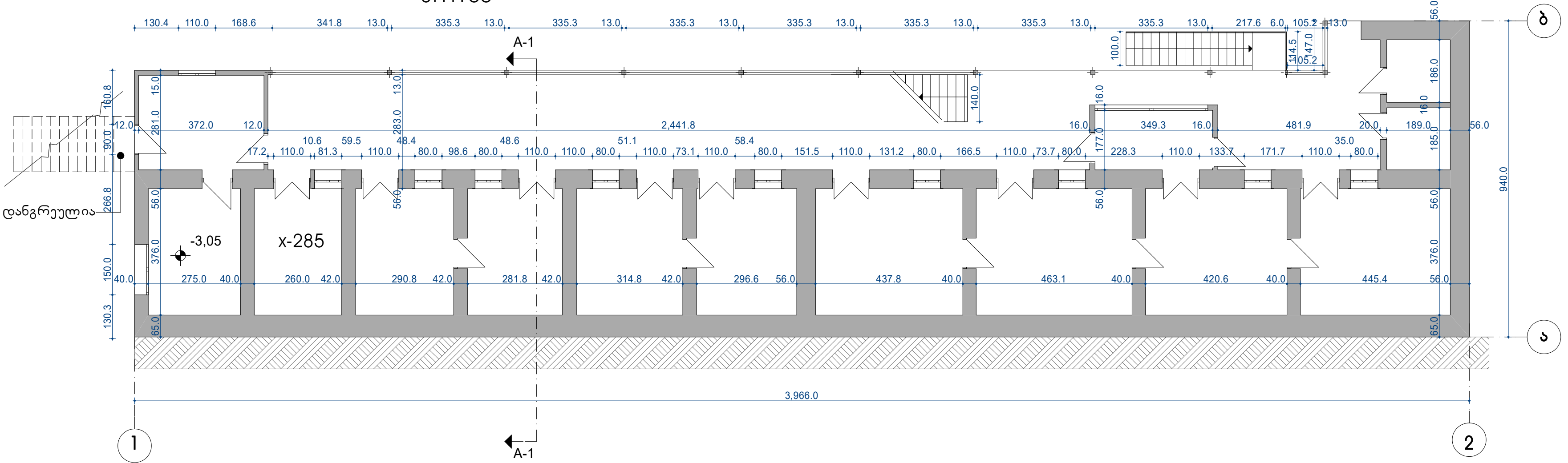
სართულის გეგმა -3,05 ნიშნულზე (ანაზომი) შ.1:100
