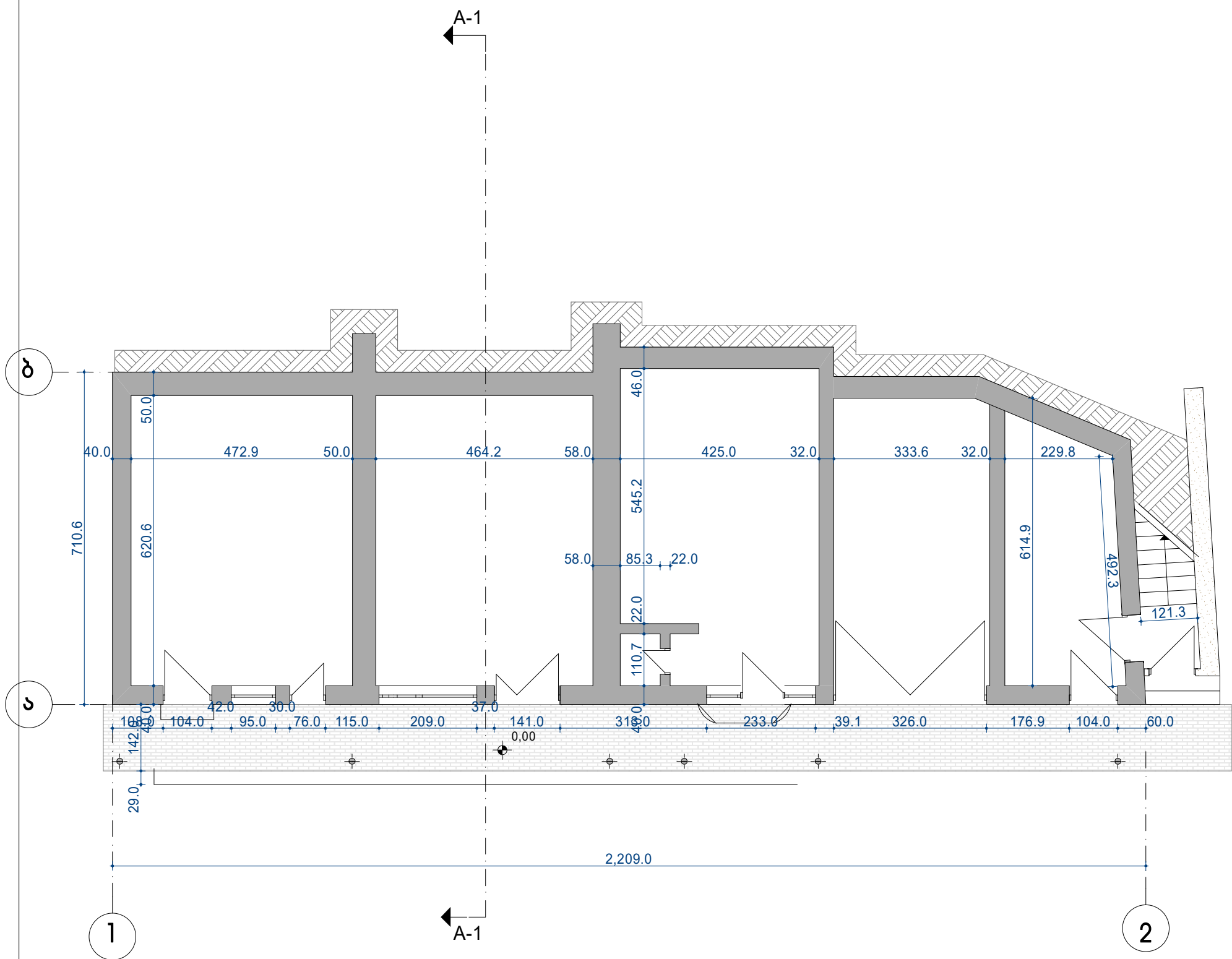
სართულის გეგმა 0,00 ნიშნულზე (ანაზომი) 8.1:100
