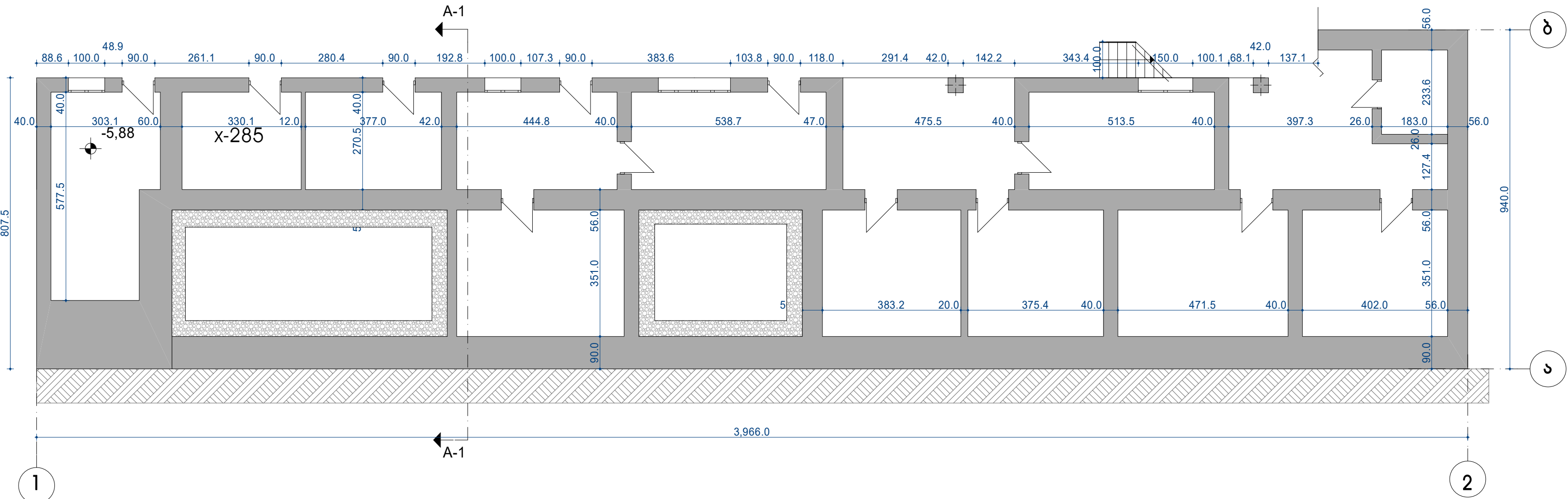
სახურავის გეგმა (ანაზომი) შ.1:100
