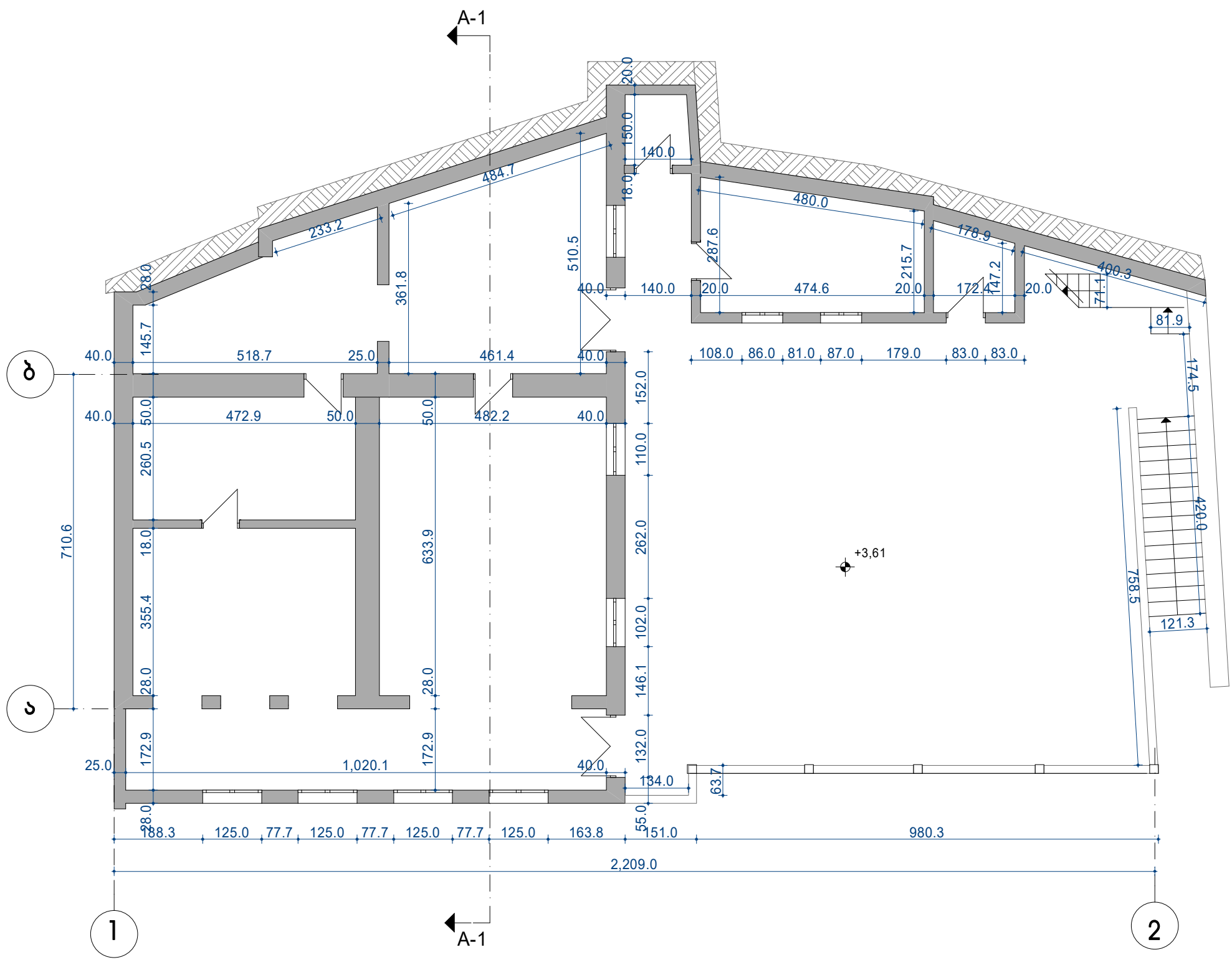
სართულის გეგმა +3,61 ნიშნულზე (ანაზომი) 8.1:100
