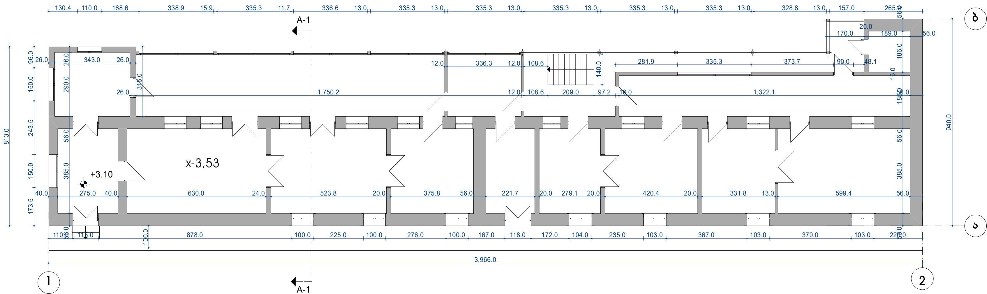
სართულის გეგმა 0,00 ნიშნულზე (ანაზომი) შ.1:100
